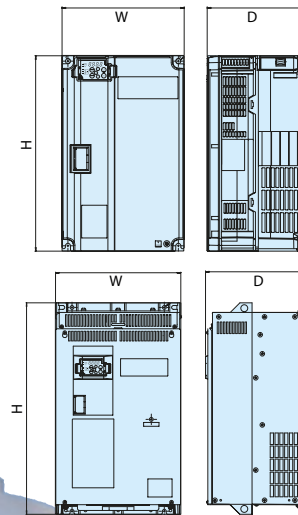
Dimensiones
